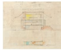
112 Oscar Tenreiro Museo del Petróleo - Cabimas , Ca. 1981 Grafito y creyón s/papel, 50 x 77 cm Firmado Precio Estimado: Bs. 850.000 - 950.000
